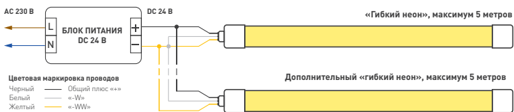
Схема 1. Прямое подключение «гибкого неона» к блоку питания (без управления оттенком)
