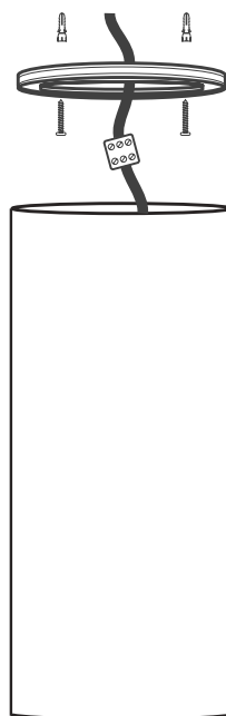
Рис. 2. Установка и подключение светильника
