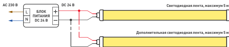
Рис. 1. Подключение нескольких светодиодных лент «неон» с одной стороны
