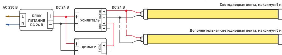
Рис. 2. Подключение светодиодных лент «неон» с возможностью изменения яркости
